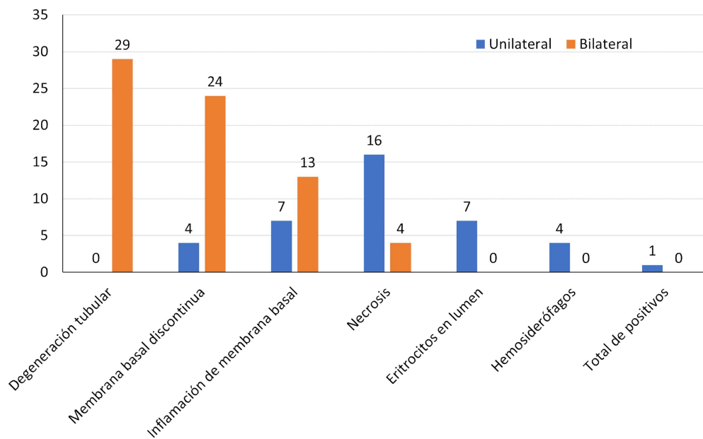
Figura 2. Lesiones histopatológicas encontradas a nivel testicular en caninos vagabundos positivos a brucelosis canina de un sector de la ciudad de Talca, Chile
