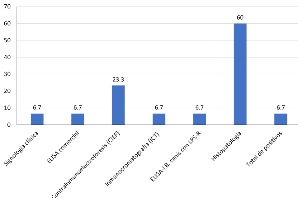
Figura 1. Frecuencia porcentual de caninos vagabundos positivos a brucelosis canina de un sector de la ciudad de Talca, Chile, según el criterio diagnóstico utilizado
