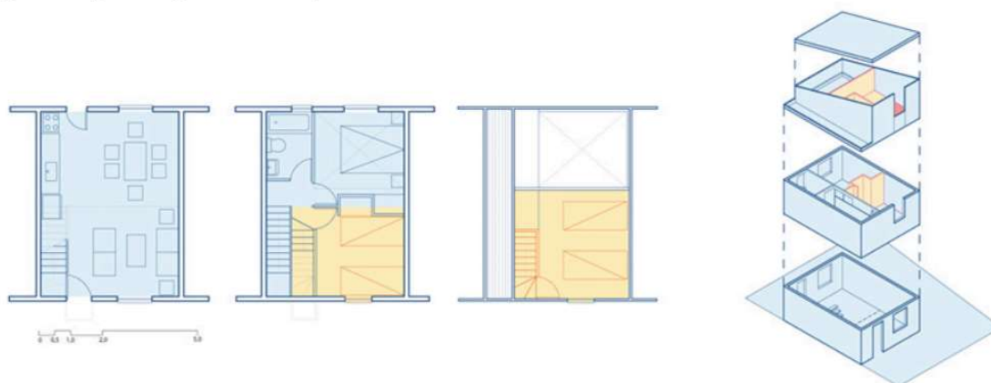
Figura 4. Etapa II, correspondiente a lo proyectado. Isométrica de la vivienda con las modificaciones propuestas por la oficina de arquitectura.
