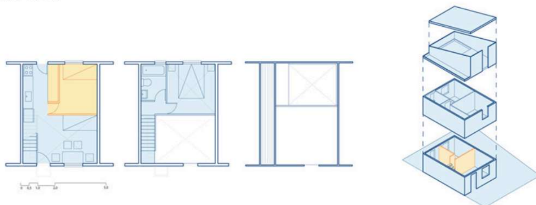
Figura 3. Etapa I, correspondiente al estado original. Isométrica de vivienda tipo entregada el año 2010.
